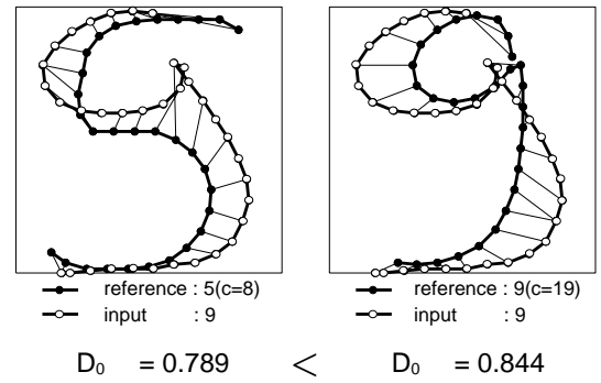
図1 合わせ過ぎによる誤認識された文字の例． Fig.1 Example of overfitting.
