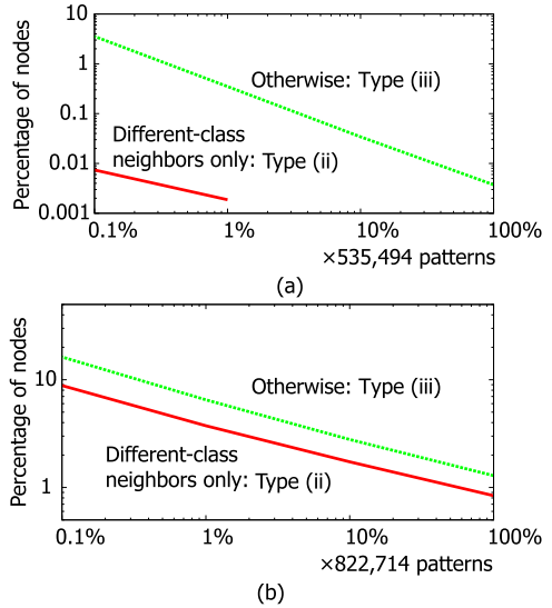
図 7 タイプ (ii) とタイプ (iii) の各ノードの割合. (a) Dataset 1 (活字), (b) Dataset 2 (手書き文字) Fig. 7 Percentage of nodes of Types (ii) and (iii). (a) Dataset 1 (machine-printed patterns), (b) Dataset 2 (handwritten patterns).
