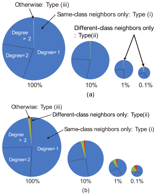
図 6 隣接ノードのクラスラベルによる分類を行ったときの各ノードの割合. (a) Dataset 1 (活字), (b) Dataset 2 (手書き文字) Fig. 6 Classification of nodes by their class consistency. (a) Dataset 1 (machine-printed patterns), (b) Dataset 2 (handwritten patterns).
