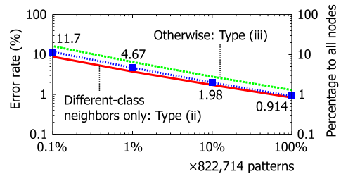
図 8 Dataset 2 (手書き文字) におけるパターン数と誤認識率、タイプ (ii) とタイプ (iii) の各ノードの割合の関係
